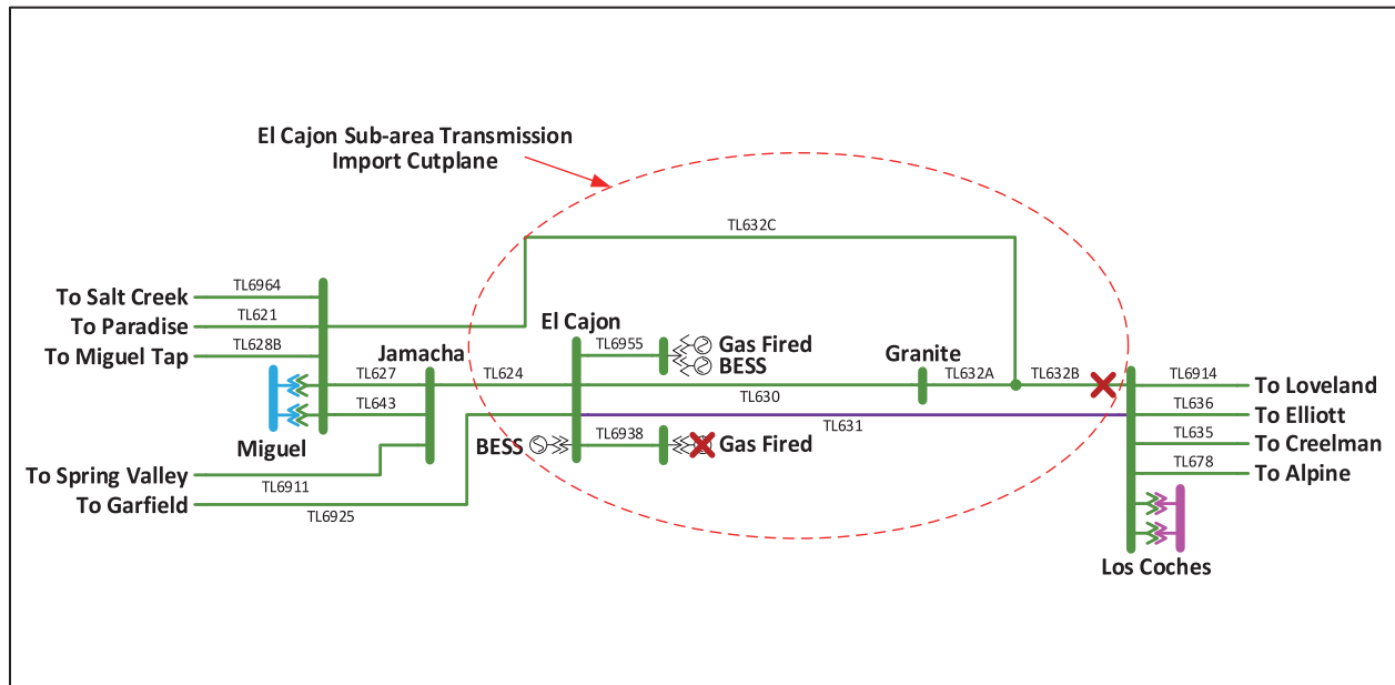
Figure 3.3-93 El Cajon LCR Sub-area
